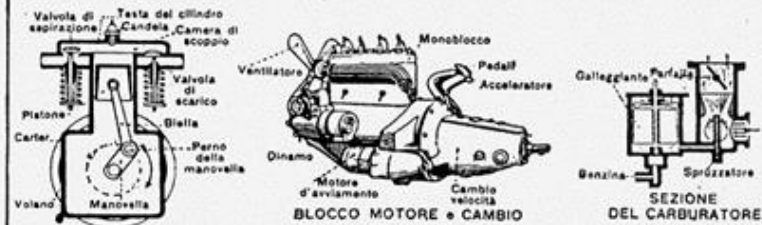
PARTI DEL MOTORE
