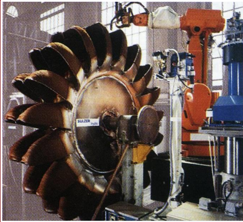
Robot trabaja sobre turbina Pelton
